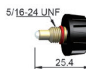
Valve Stem 阀杆
