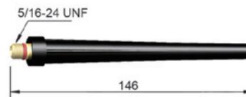
Long Back Cup 长压帽
